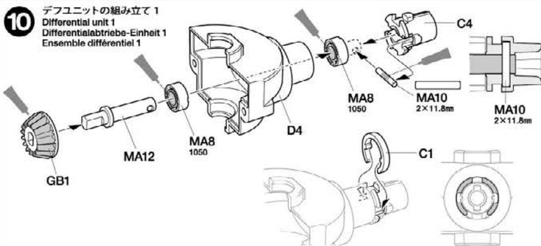
MA8 ×2 1050プラベアリング Plastic bearing Plastik-Lager Palier en plastique
