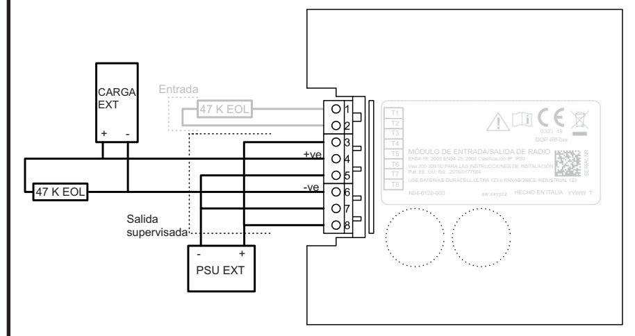
Figura 6: Módulo de salida supervisado
