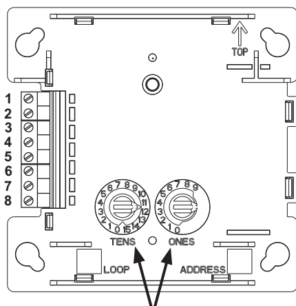
Abb. 5: Vorderseite des Moduls mit Adressschaltern
