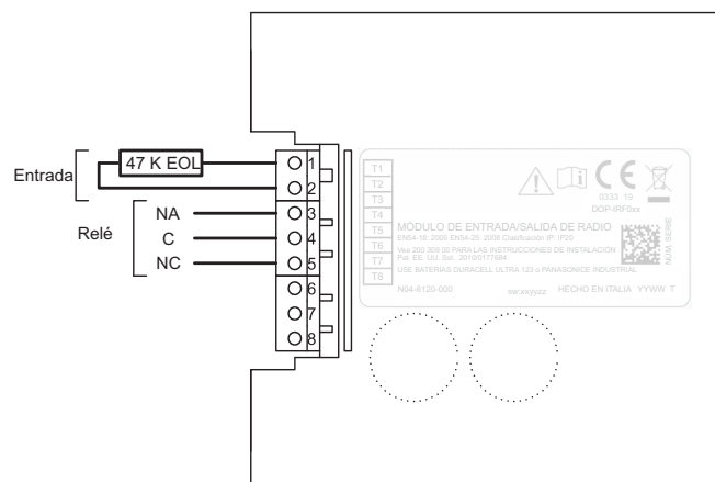
Figura 7: Modo de relé del módulo de entrada/salida
