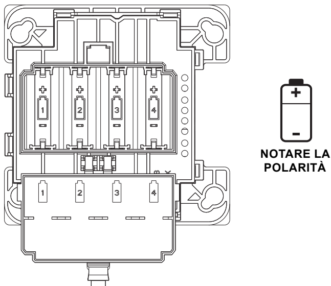
Figura 5: Parte anteriore del modulo con interruttori indirizz
