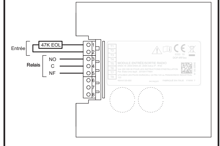
Figure 7 : Mode relais du module entrée/sortie
