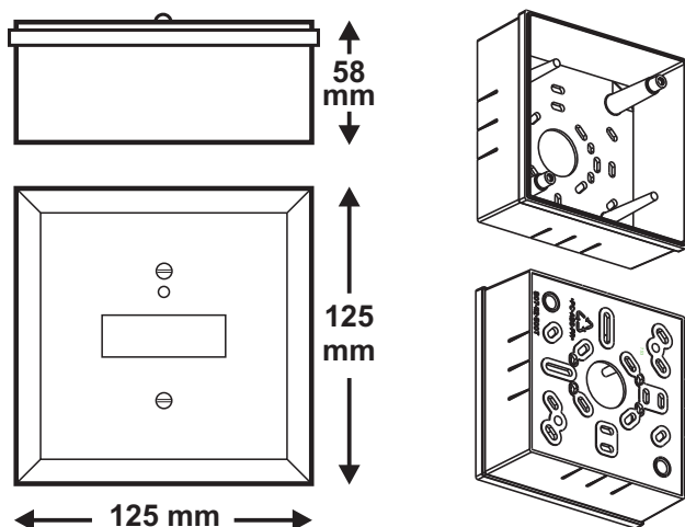
Figura 1: Dimensioni esterne modulo IO + scatola posteriore
