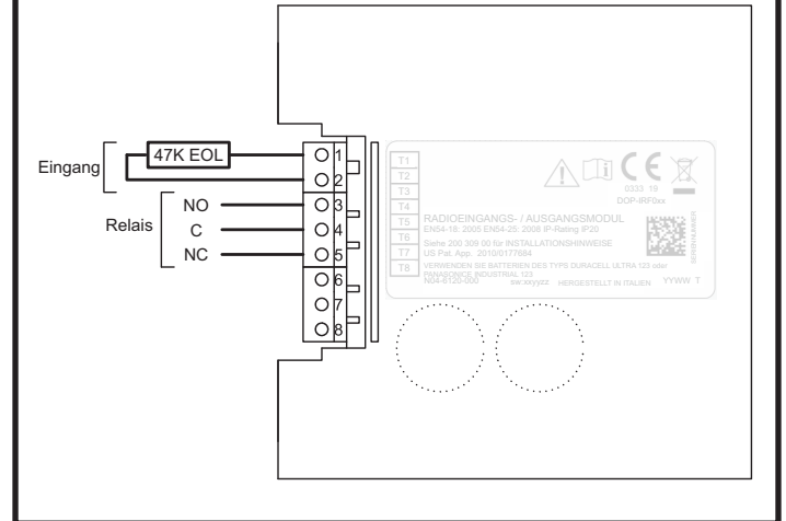
Abb. 7: Eingang / Ausgangsmodul Relaismodus
