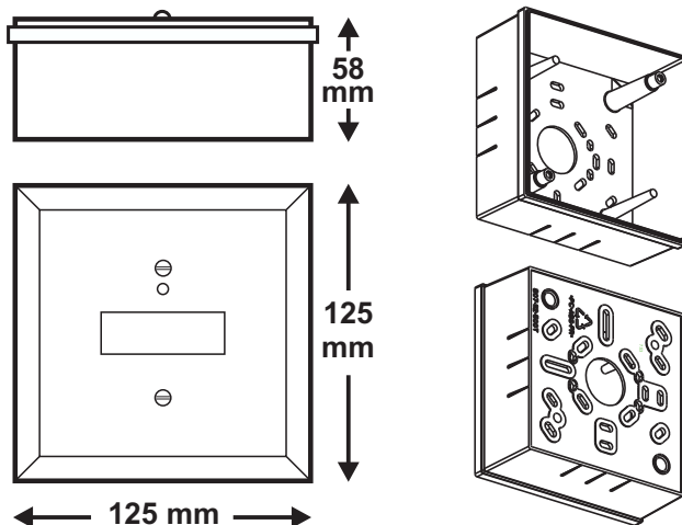
Abb. 1: IO-Modul + äußere Abmessungen der Gehäuse
