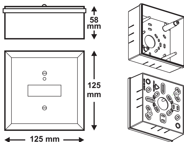
Figure 1 : Module IO + dimensions extérieures du boîtier arrière
