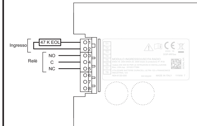
Figura 7: Modalità relè modulo ingresso/uscita
