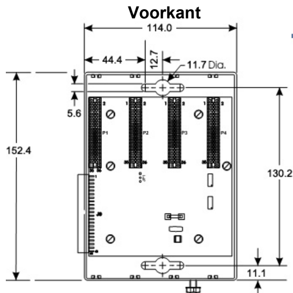
Afbeelding 3. Afmetingen (mm) uitbreidingsbehuizing ControlWave Micro met 4 sleuven
