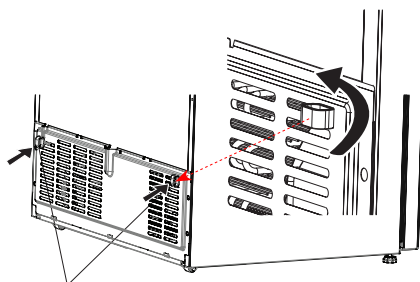
Plastic voor afstandinstelling
