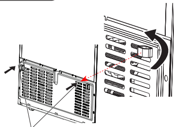
Pieza de plástico para ajustar la distancia entre la pared trasera y el frigorífico
