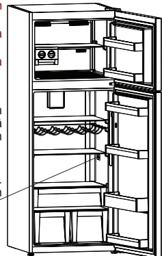
Lämpötilasensorin alue
