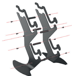
Fig 1. Ilustración de montaje.
