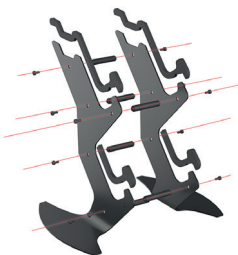
1. att. Montāžas ilustrācija.
