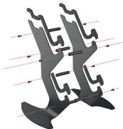
Fig 1. Afbeelding van montage.
