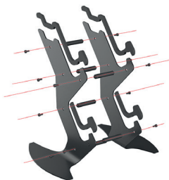
Figur 1. Monteringsillustrasjon.
