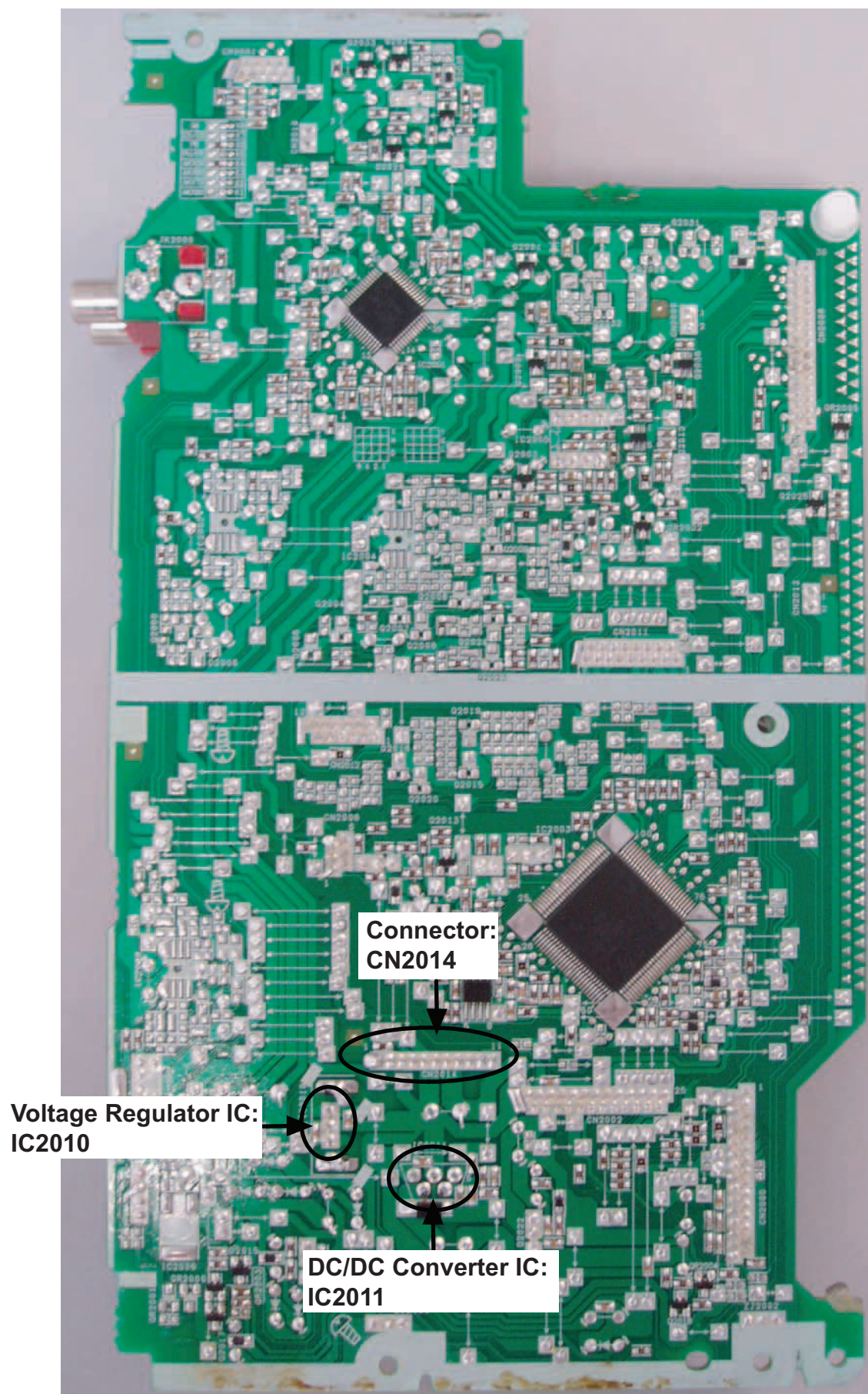
Fig. 2 Main P.C.B.
