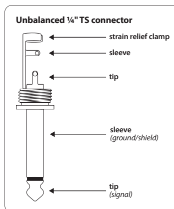
Fig. 2.2: Connettore jack TS da ¼"
