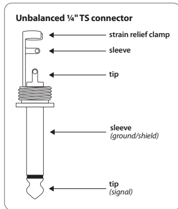
Abb. 2.3: ¼" TS Boxenanschluss
