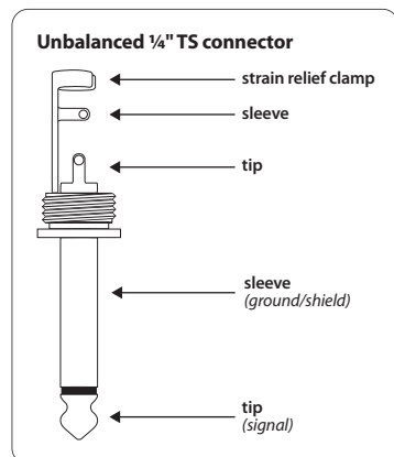
Fig. 2.2: Connecteurs Jacks 6,35 mm mono
