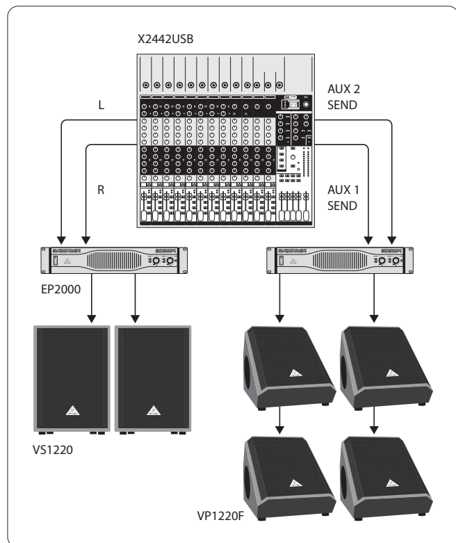
Fig. 5.2: Fullständig stereofunktion med golvmonitorer
