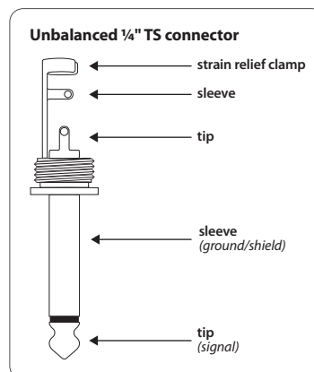
Fig. 2.2 : 1/4" TS luidsprekerconnector
