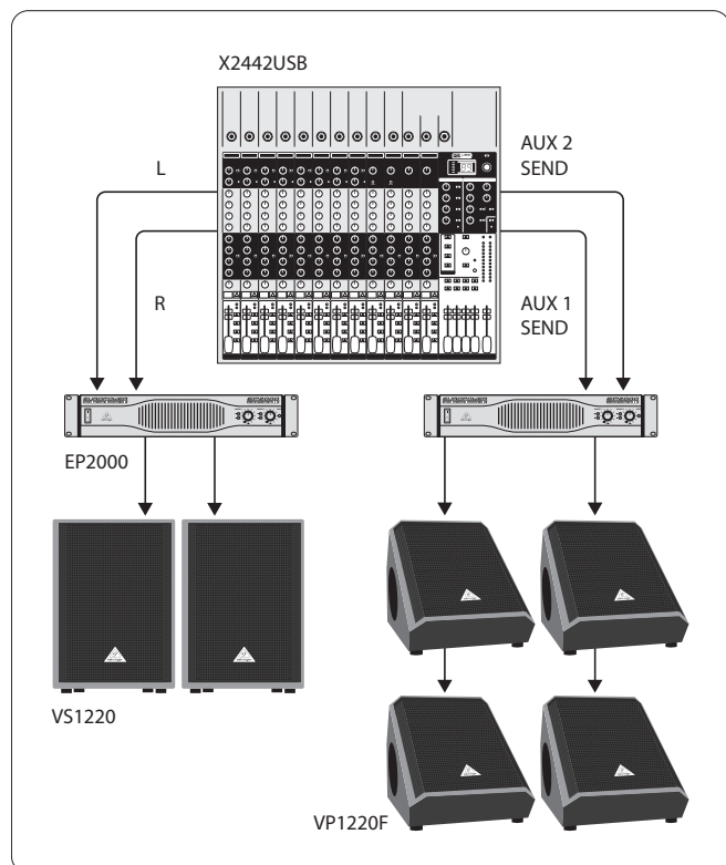
Fig. 5.2: Tryb pracy monitorów scenicznych w układzie stereo i w pełnym paśmie częstotliwości
