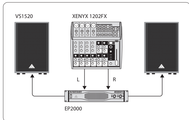
Fig. 5.1: Operação em estéreo com full-range
