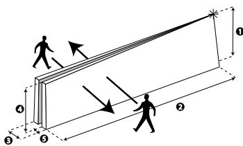
Figure 25. Schéma du rayon de détection
