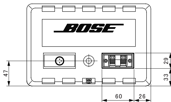
A矢視図
