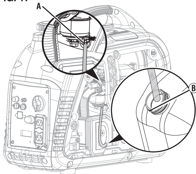
A - Válvula de drenaje B - Manguera de drenaje
