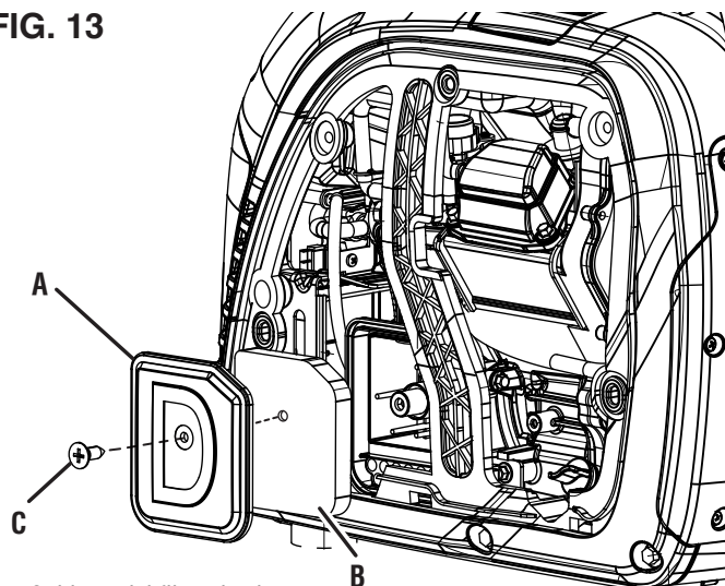
A - Cubierta del filtro de aire B - Filtro de aire C - Tornillo
