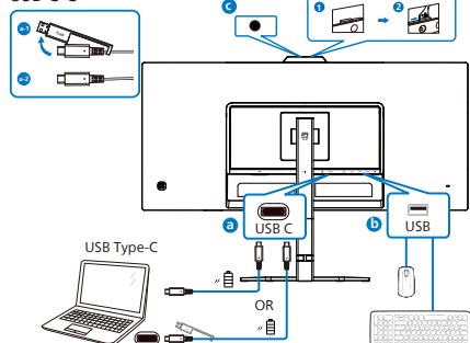
USB C-C
