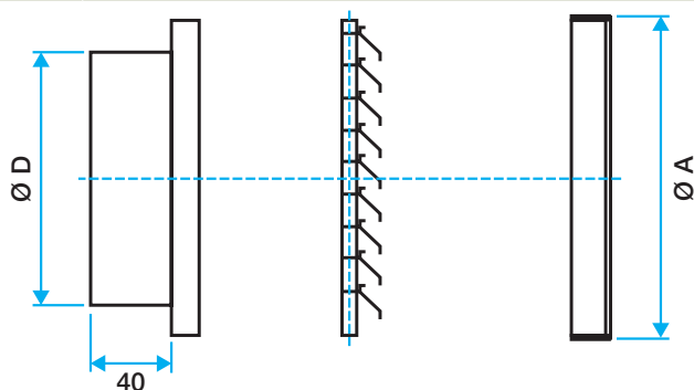
Grille AR 637 diamètre 125 à 315 mm
