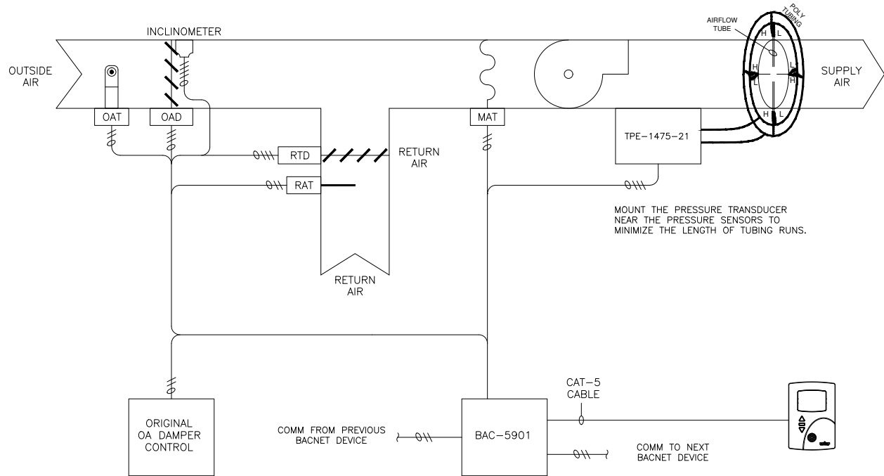
AFMS LAYOUT
