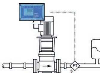
Schema di regolazione pompe basato sulla misura di portata
