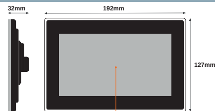
Display 7" 800 x 480 pixel, tecnologia TFT, 16M colori
