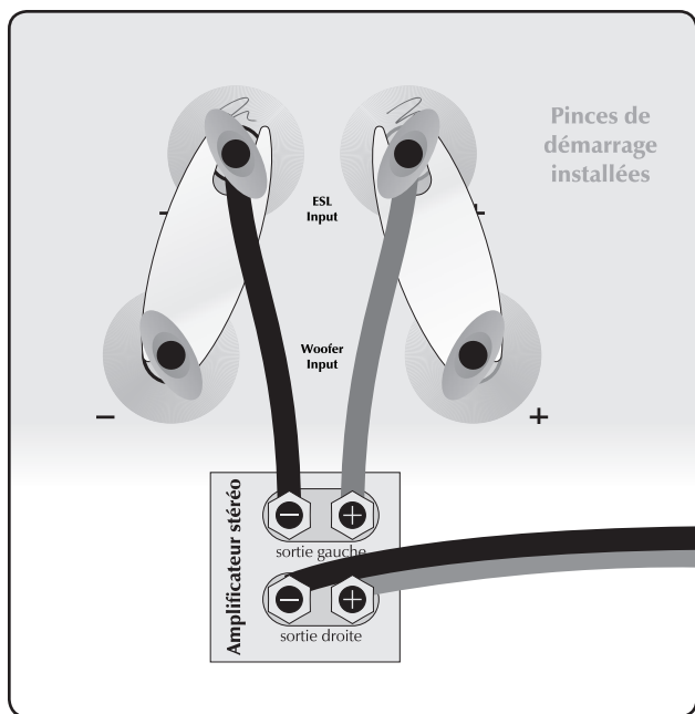
Raccord à un fil. Un canal illustré.
