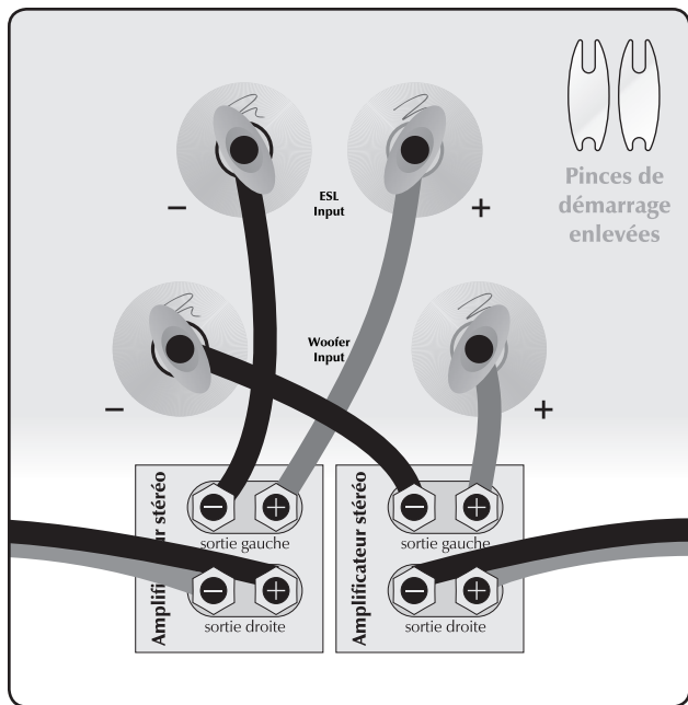
Raccordement par bi-amplification horizontale. Un canal illustré.
