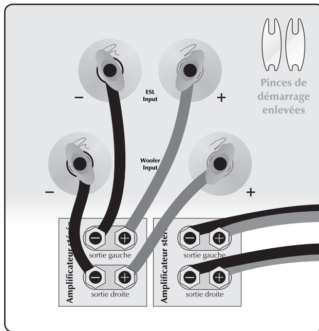
Raccordement par bi-amplification verticale. Un canal illustré.
