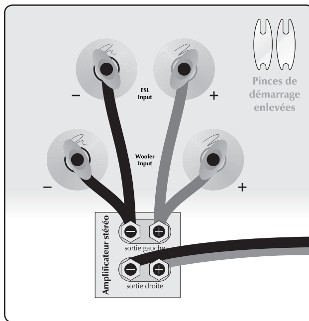
Raccord à deux fils. Un canal illustré.
