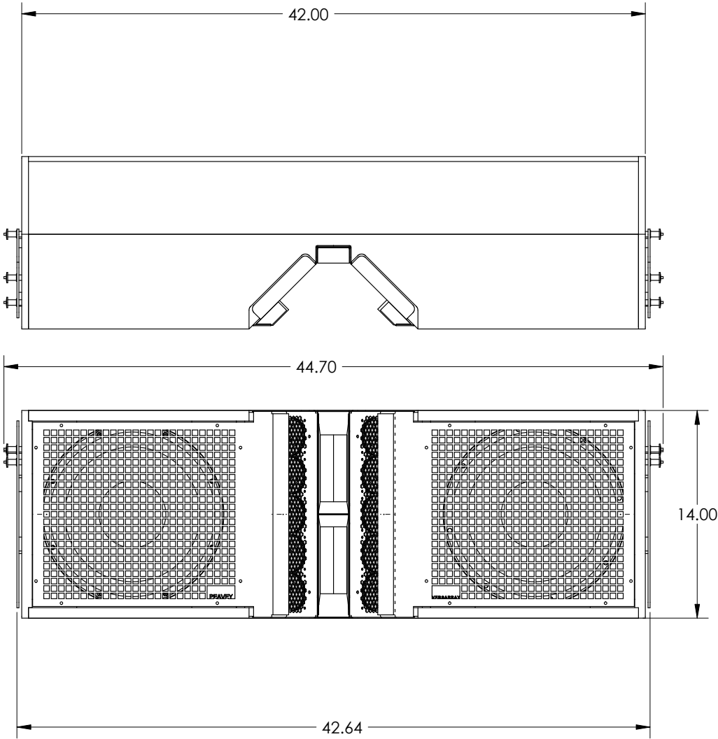
Versarray™ 212 Cabinet Dimensions
