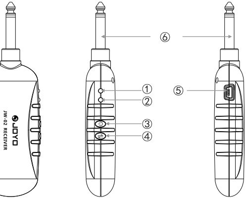
接收器示意
