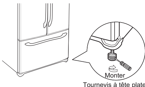
Tournevis à tête plate
