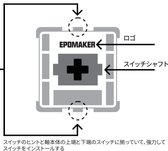
スイッチのピンと軸本体の上端と下端のスイッチに揃って、強力してスイッチをインストールする
