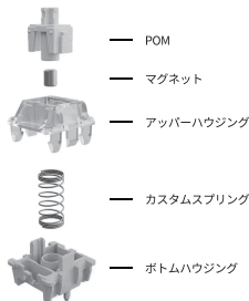
スイッチのピンと軸本体の上端と下端のスイッチに揃って、強力してスイッチをインストールする
