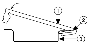
Figure 37. DIN Rail Clip Parts Locator
