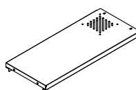
Panneau gauche du compartiment supérieur x 1
