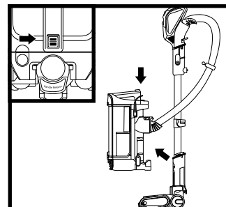
PROPULSIÓN LIFT-AWAY®
