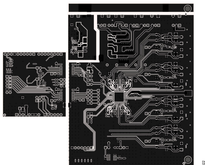
Figure 24. EVAL-AD74416H-ARDZ Layer 1, Top Layer
