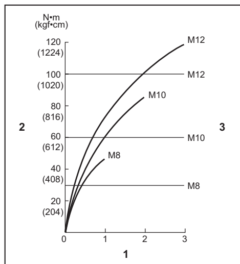
1. Aandraaitijd (seconden) 2. Aandraaimoment 3. Juiste aandraaimoment afhankelijk van de boutdiameter
