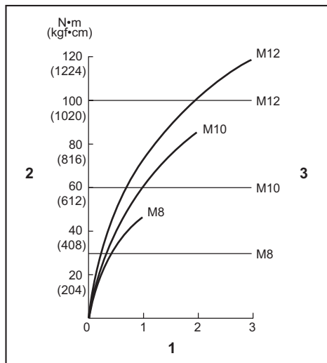
1. Durée de serrage (en secondes) 2. Couple de serrage 3. Couple de serrage correct correspondant à chaque diamètre de boulon
