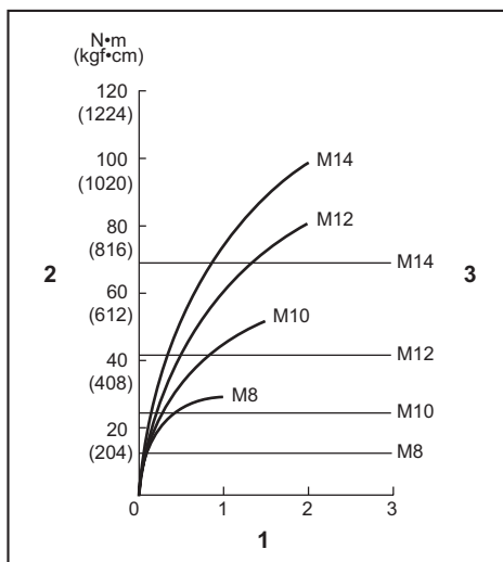
1. Tempo de aperto (segundos) 2. Binário de aperto 3. Binário de aperto adequado correspondente ao diâmetro de cada perno
