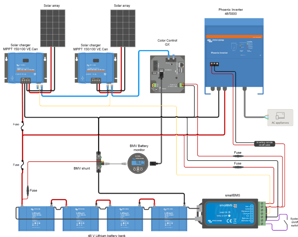
Illustration 4 : application solaire avec deux MPPT 150/85 avec un bus CAN.
