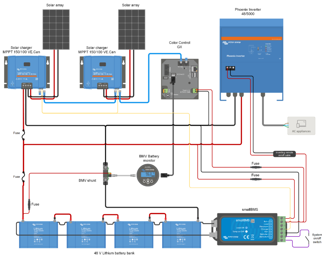
Abbildung 4: Solaranlage mit zwei MPPT 150/85 Can-bus.
