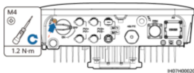
Figura 4-16 Instalación del tornillo de bloqueo del interruptor de CC
