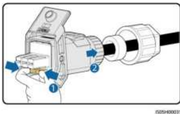
Figura 5-12 Extracción de un accesorio de inserción
