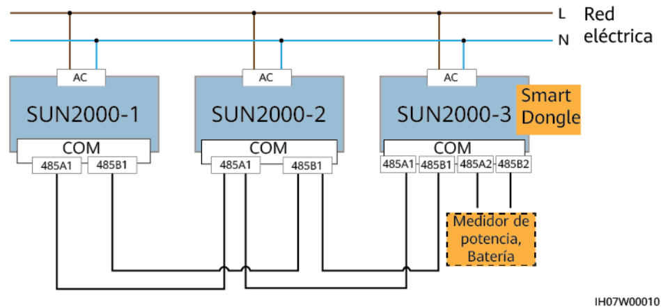
Figura 5-21 Conexión a la red en fase
