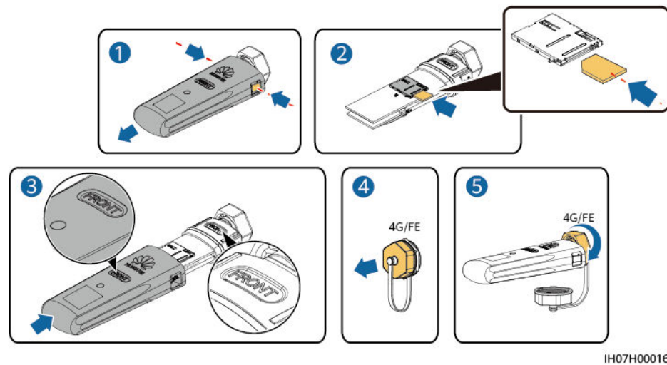
Figura 5-4 Instalación de un Smart Dongle 4G
