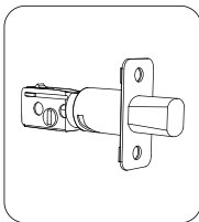
f. Deadbolt
