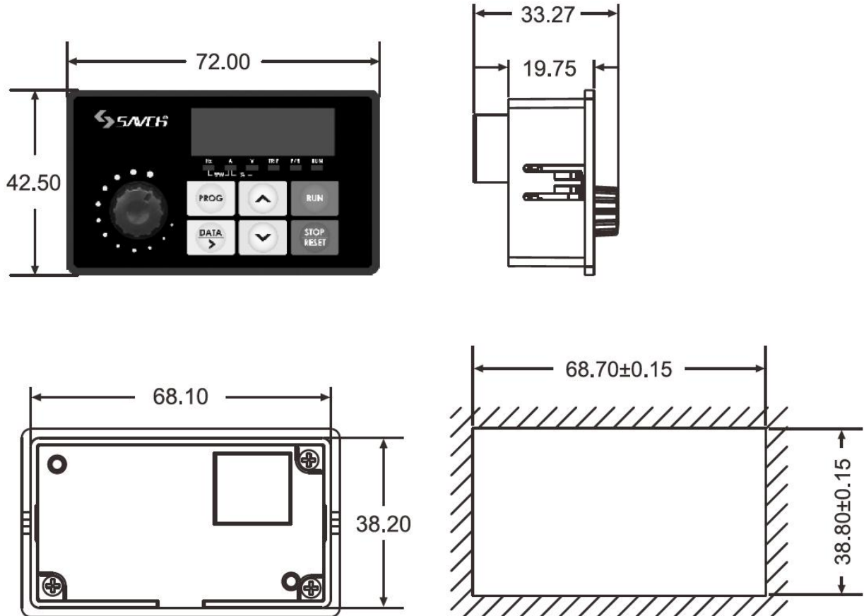
Keypad dimensions
