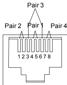
T568B
