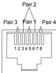
T568A
