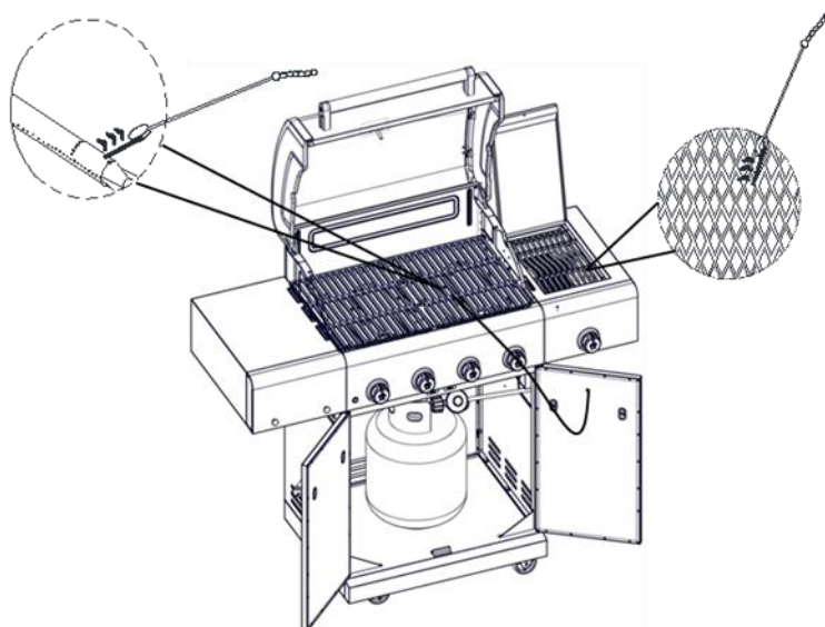
Quemador principal
