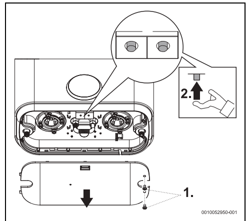
Fig. 16 Termostatos de seguridad
