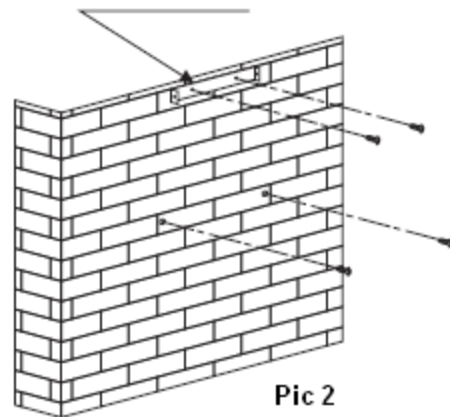
Indvendigt skaktsbeslag
