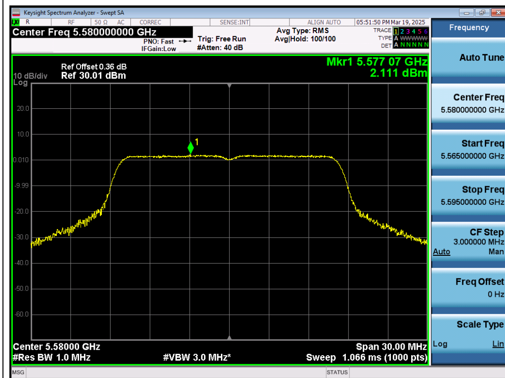
Test_Graph_802.11a_ANT1_5580_6Mbps_PSD
