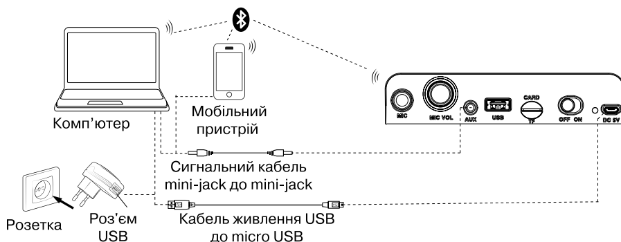
Мал. 3. Схема підключення
