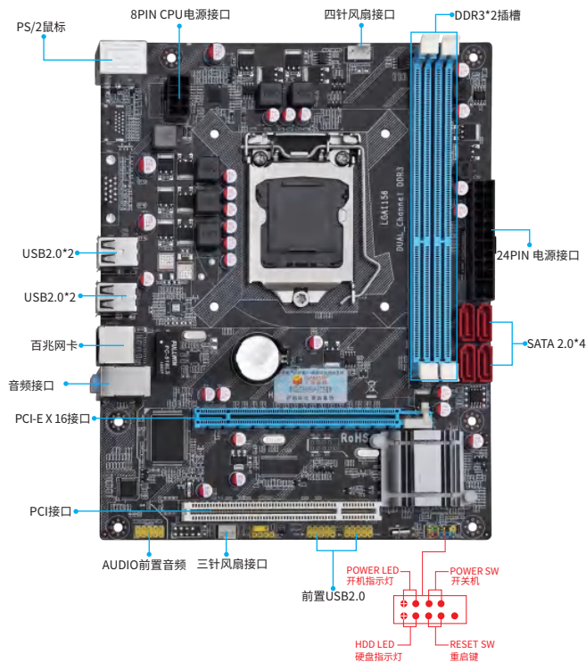
图1-1 P55主板图解
