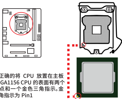
图2-7 CPU安装
