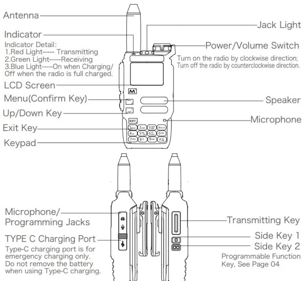
Figure 1 : Les différentes commandes du QUANCHENG UV-K5 (Doc. Quansheng)
