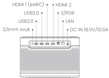
Zpětný pohled
