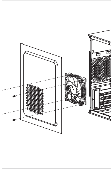
(6c) Install Side Fan
