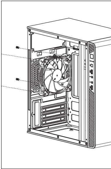
(6b) Install Rear Fan
