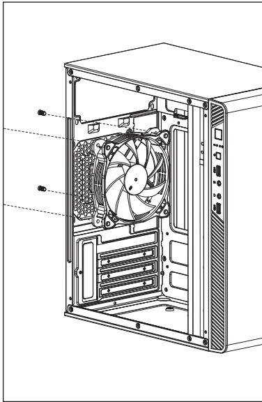
(6b) Install Rear Fan
