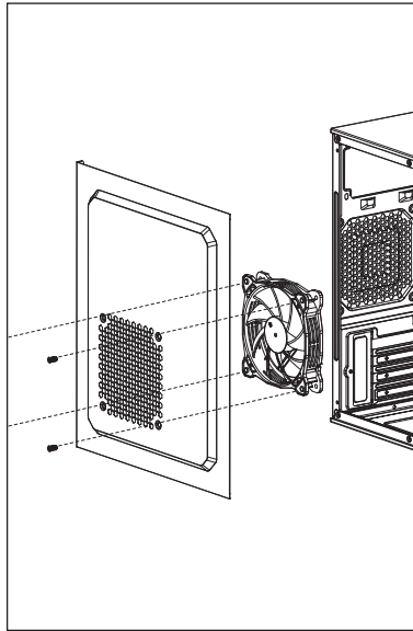
(6c) Install Side Fan
