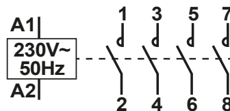
SC-101-2P-25-40 (4NO)
