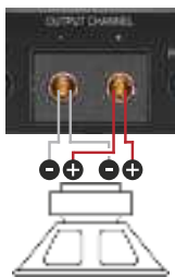
Ein Subwoofer mit Doppelschwingspule (Dual Voice Coil)
