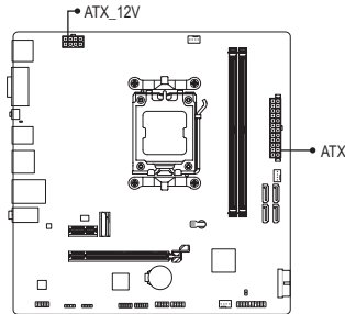
ATX_12V:
