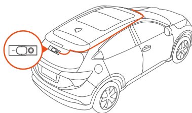
⑥ リアカメラのケーブルの配線
