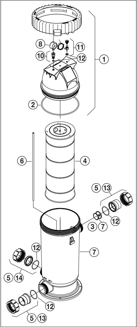
Figura 7. Diagrama ampliado de CS Series
