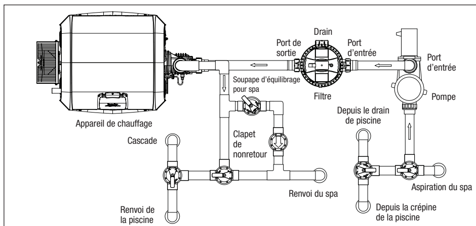
Figure 3. Plomberie basique pour combinaison piscine/spa
