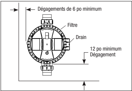
Figure 1. Emplacement du filtre - Vue de dessus
