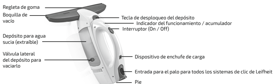
Imagen 2: elementos de control del aspirador de ventanas
