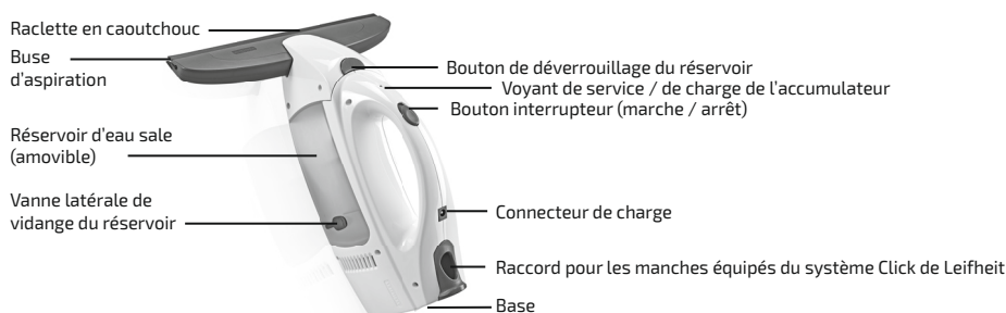
Figure 2 : Les différents composants de l'aspirateur à vitres
