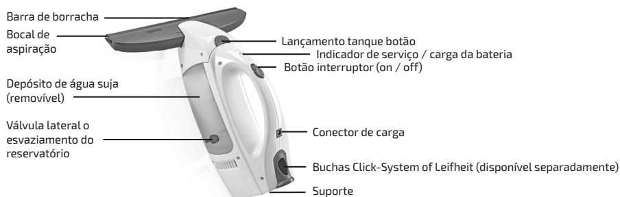
Figura 2: Os diferentes componentes do limpa-vidros
