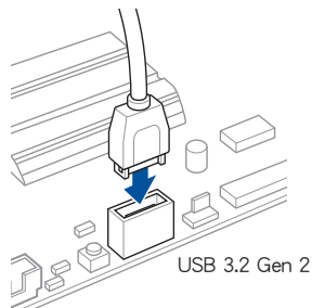
安装 USB 3.2 Gen 2 连接插槽
