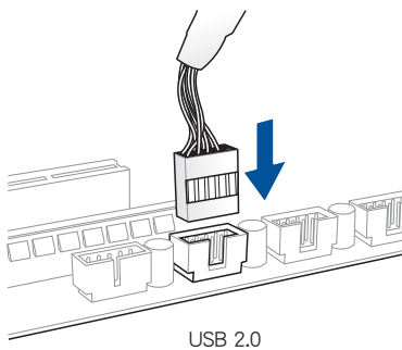
安装 USB 2.0 连接插槽
