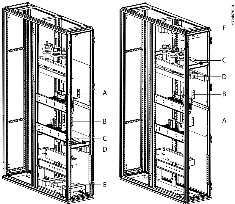
Ilustração 47: Entrada Inferior (Esquerda) e Entrada Superior (Direita)
