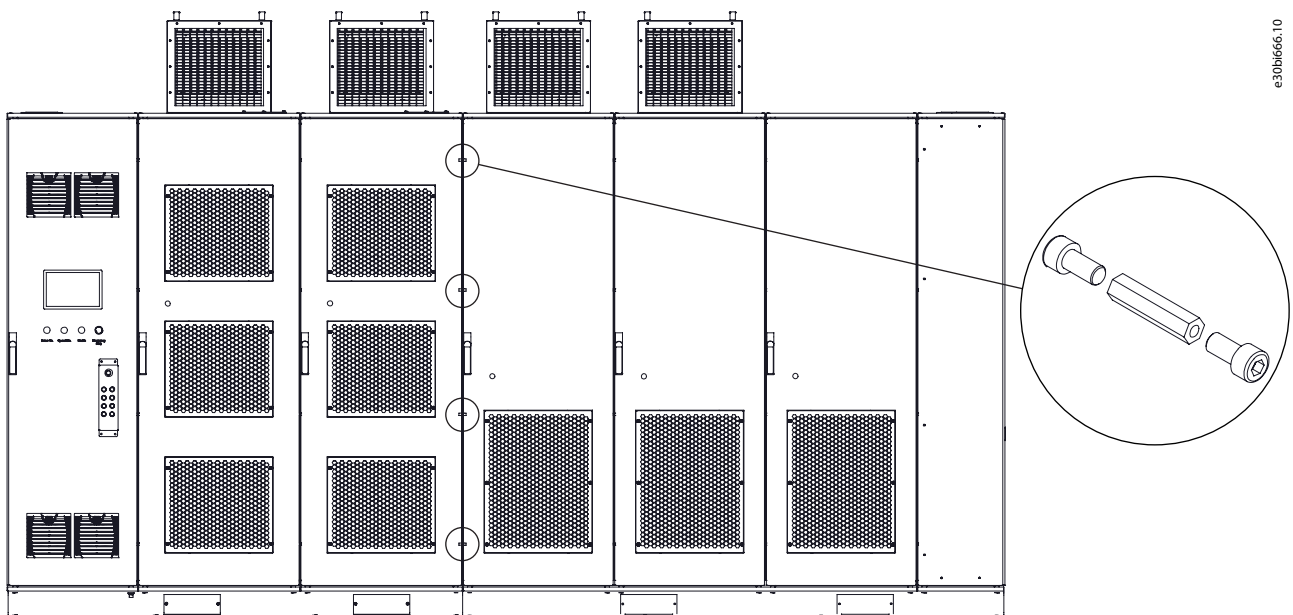
Ilustração 37: Pontos de Junção em Gabinetes Line-Up
