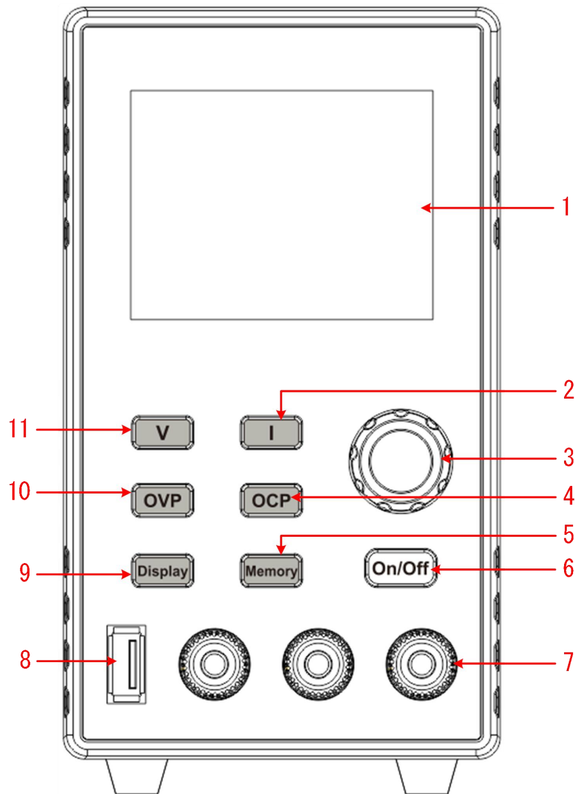
Abbildung 3- 1 Übersicht der Vorderseite
