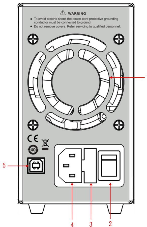
Abbildung 3-2 Übersicht der Rückseite
