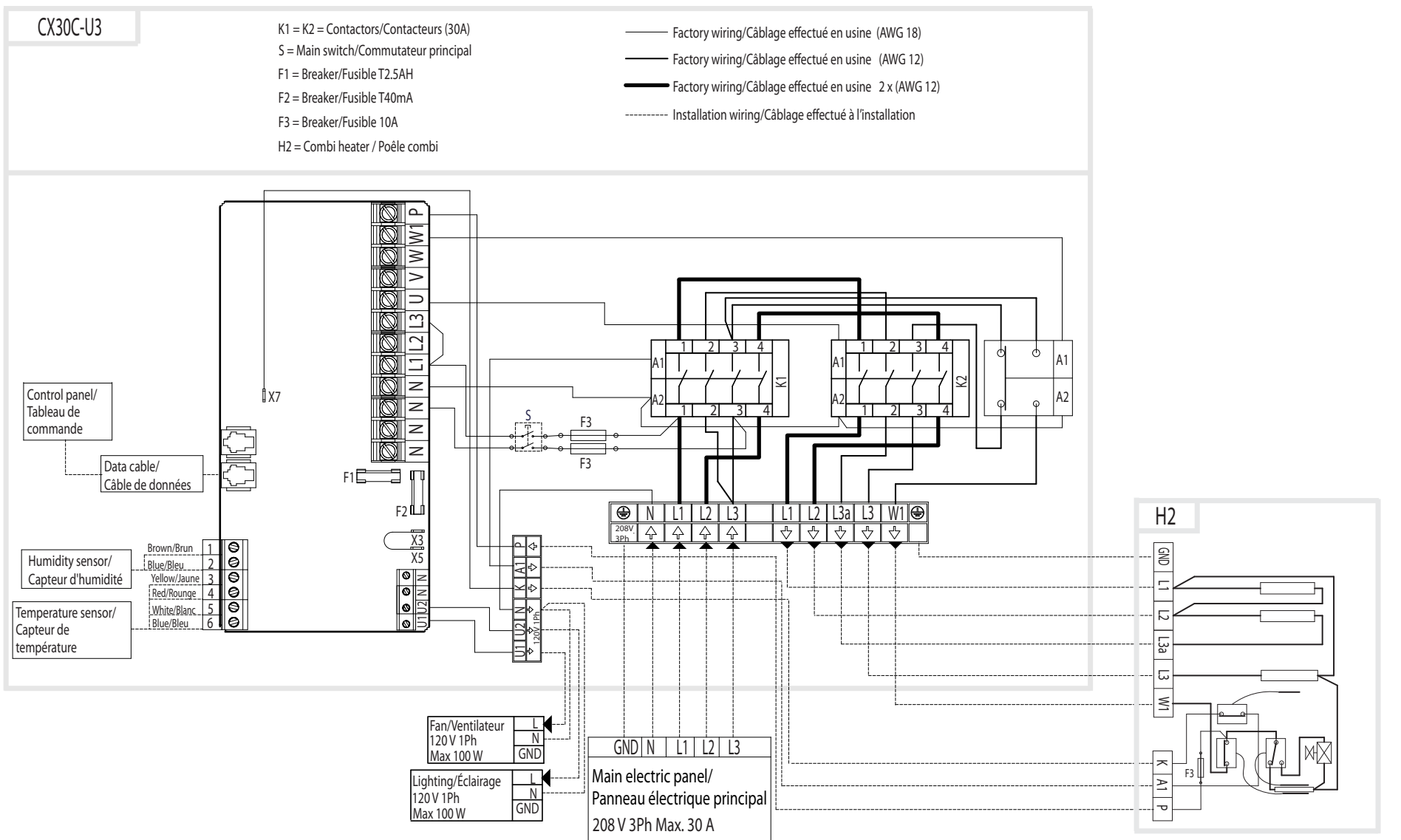
Figure 6b. Electrical connections 208 V, 3Ph (CX30C-U3). Figure 6b. Connexions électriques 208 V, 3Ph (CX30C-U3).
